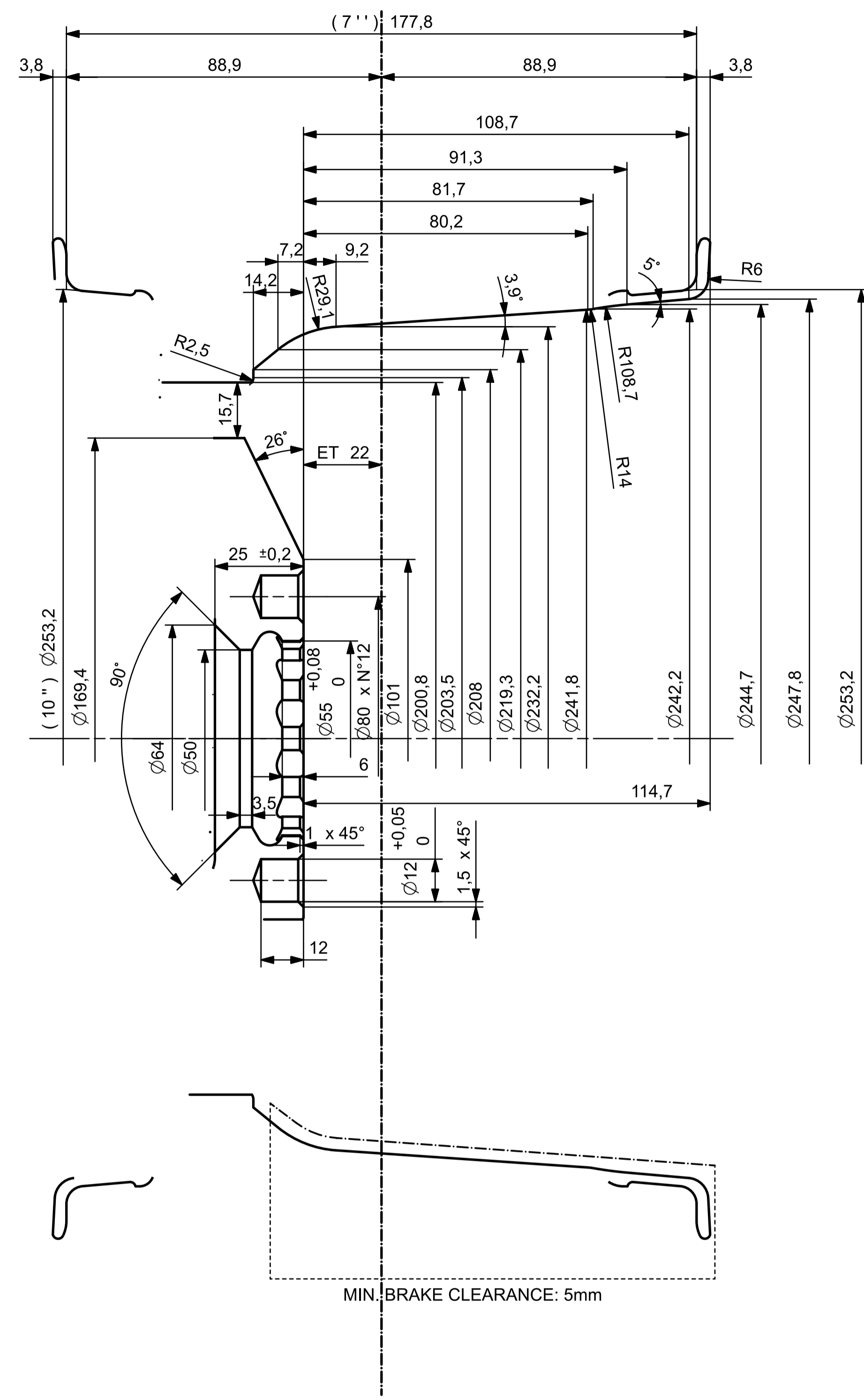
SECTION A-A
